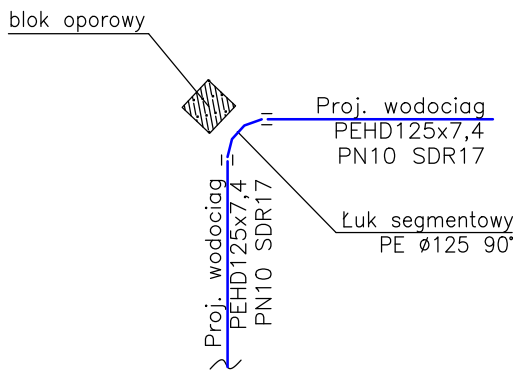
Schemat węzła nr W11
