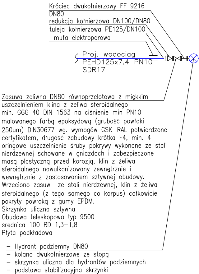
Schemat węzła nr HP1
