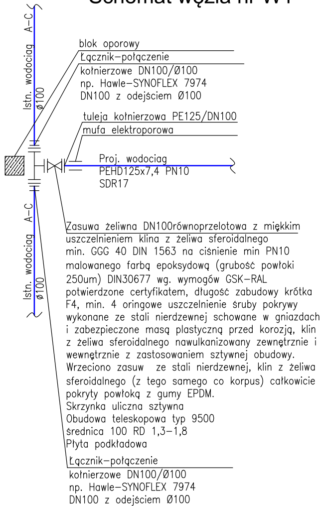
Schemat węzła nr W1
