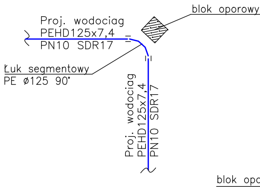
Schemat węzła nr W7
