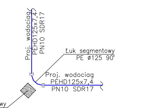
Schemat węzła nr W8
